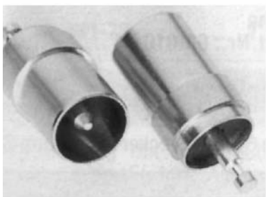
Rys. 3 Wtyk koncentryczny
